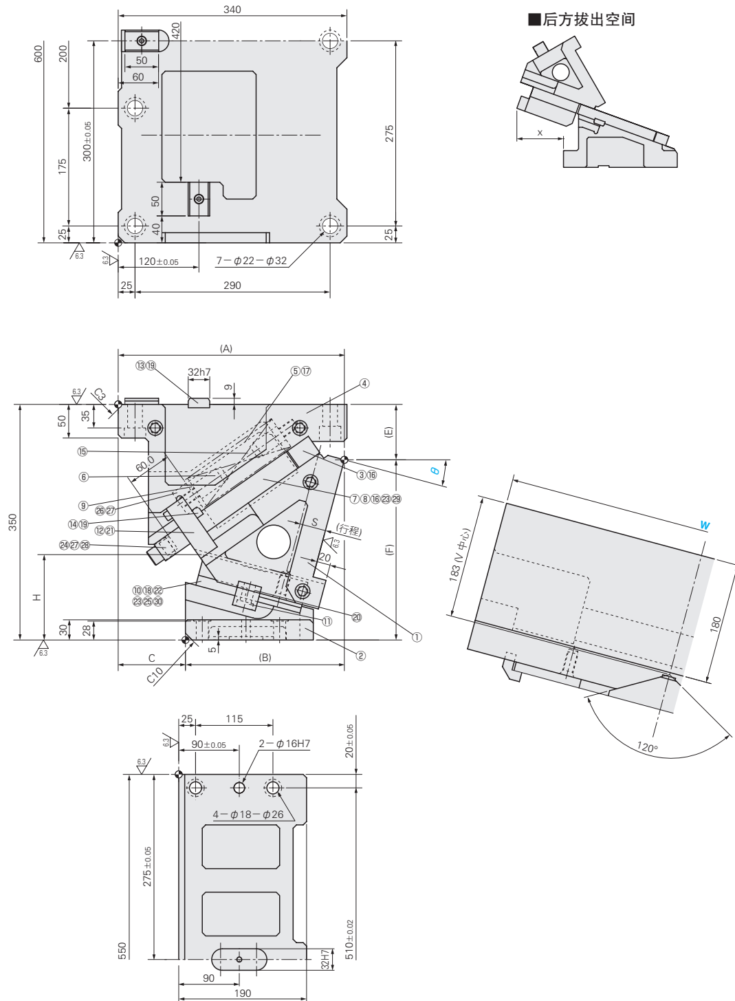
■斜楔行程关系图 P.1247
