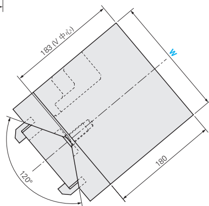
■斜楔行程关系图 P.1247
