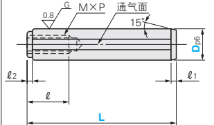
MST (带拉拔螺纹p6型)
