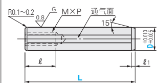
MSTP (带拉拔螺纹精密型)
