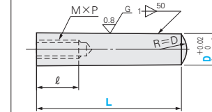
MTT (带拉拔螺纹锥型)
