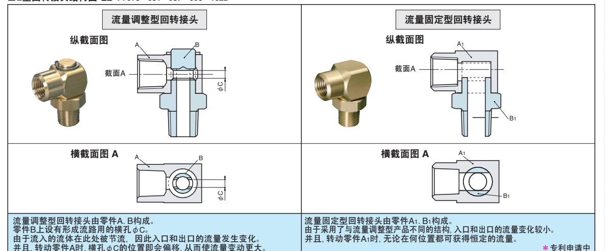
■ L型回转接头结构图 P.978·981·987·998·1022
