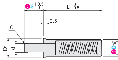
C-MPFS (平面型)
