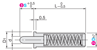
C-MPJS (球面型)
