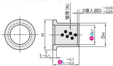
C-MUFZU (薄壁型)
