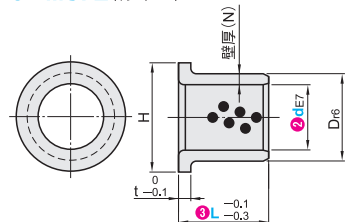
C-MUFZ (標準型)
