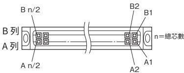
插座(母端)連結器嵌合面視圖
