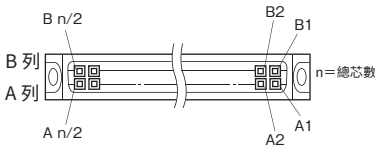
插座(母端)連結器嵌合面視圖
