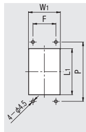
面板安裝孔尺寸
