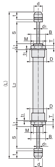
行程S 50 兩端螺牙型
