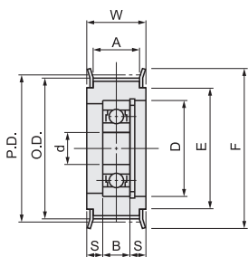
單軸承
