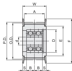
雙軸承
